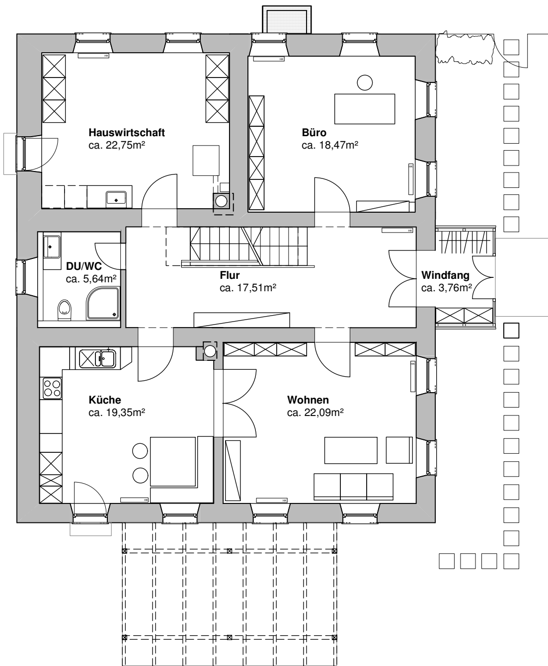
GRUNDRISS ERDGESCHOSS
