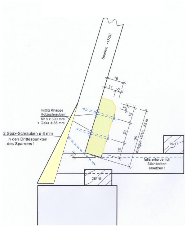
INSTANDSETZUNG TRAUFPUNKTE
