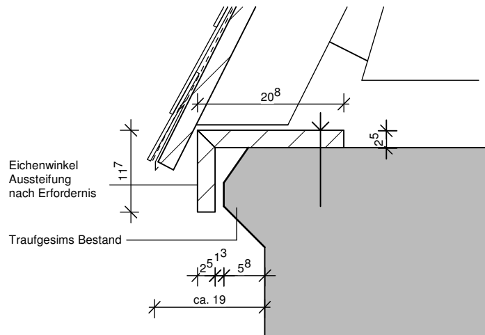
TRAUFAUSBILDUNG SÜDSEITE
